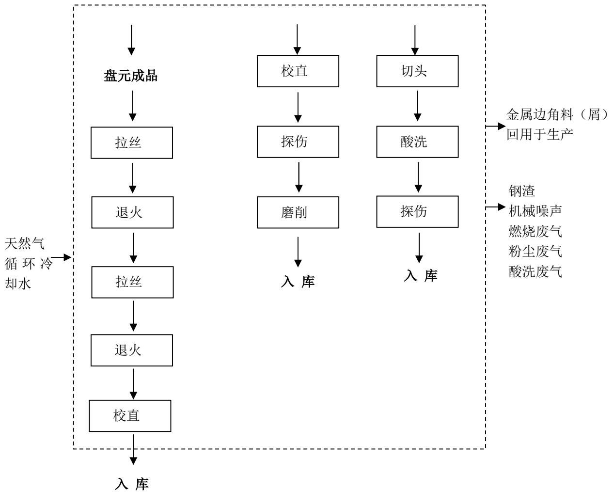
图 1 生产工艺及产污环节图
