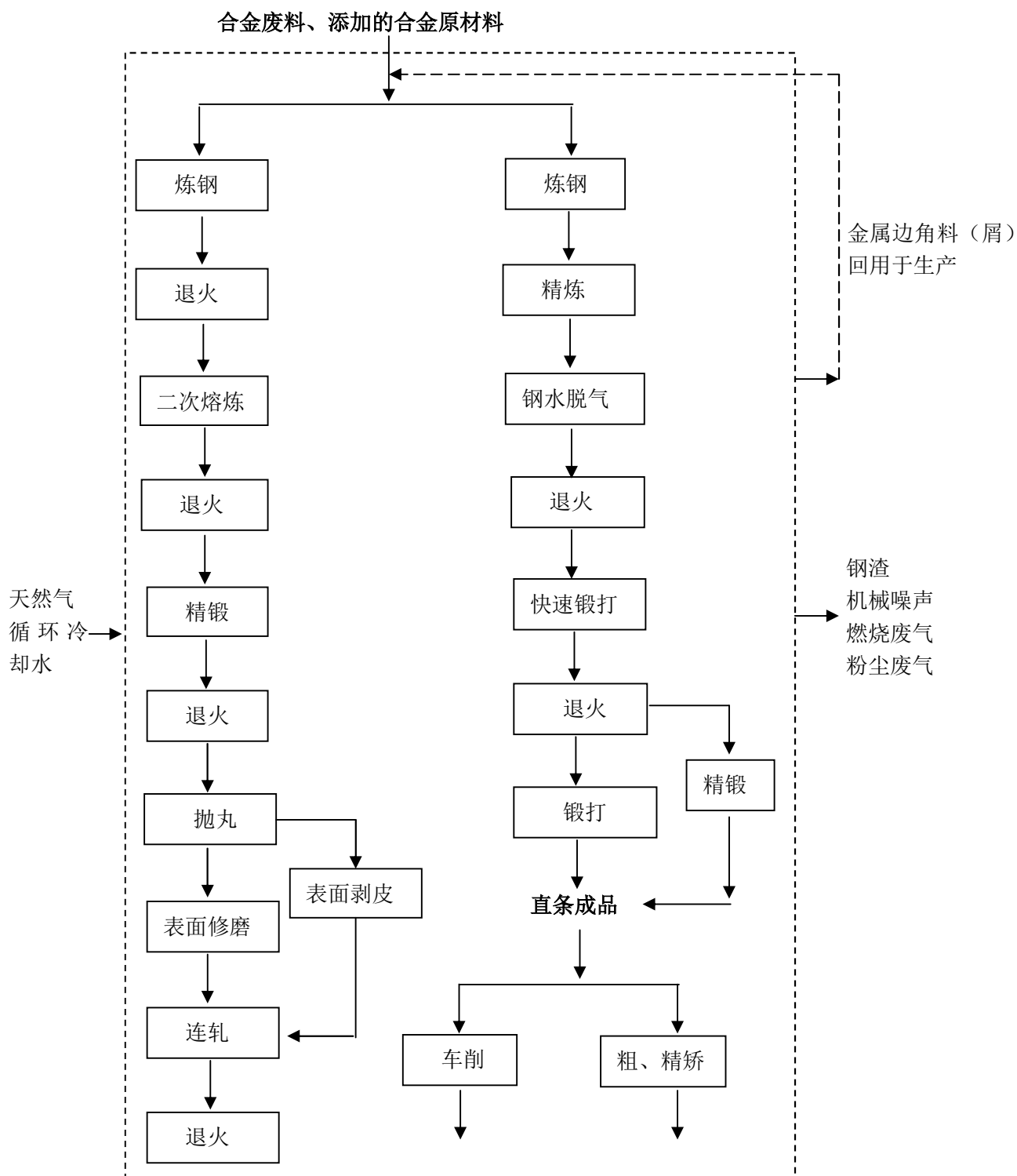
高速工具钢生产工艺及产污环节图
