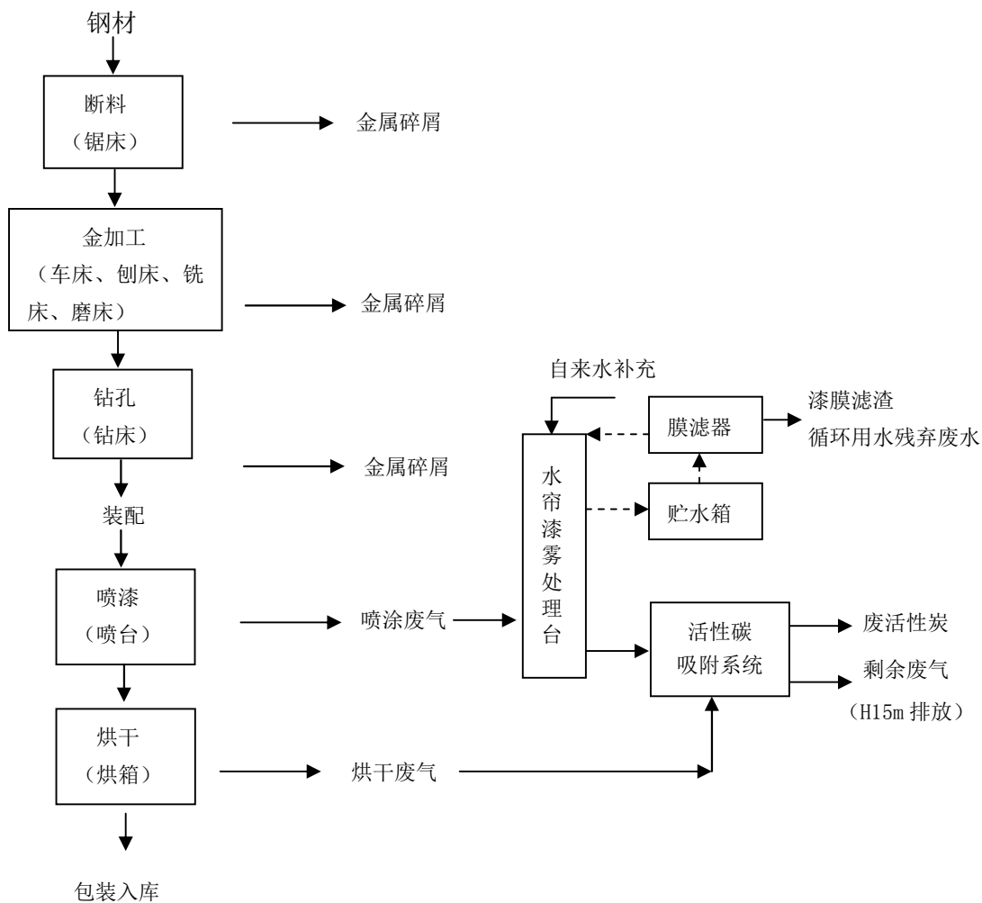
碾米机生产工艺及产污环节图
