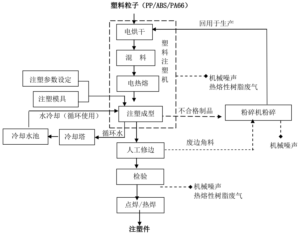
图 2.2-1 塑料件注塑成型工艺流程及产污环节图
