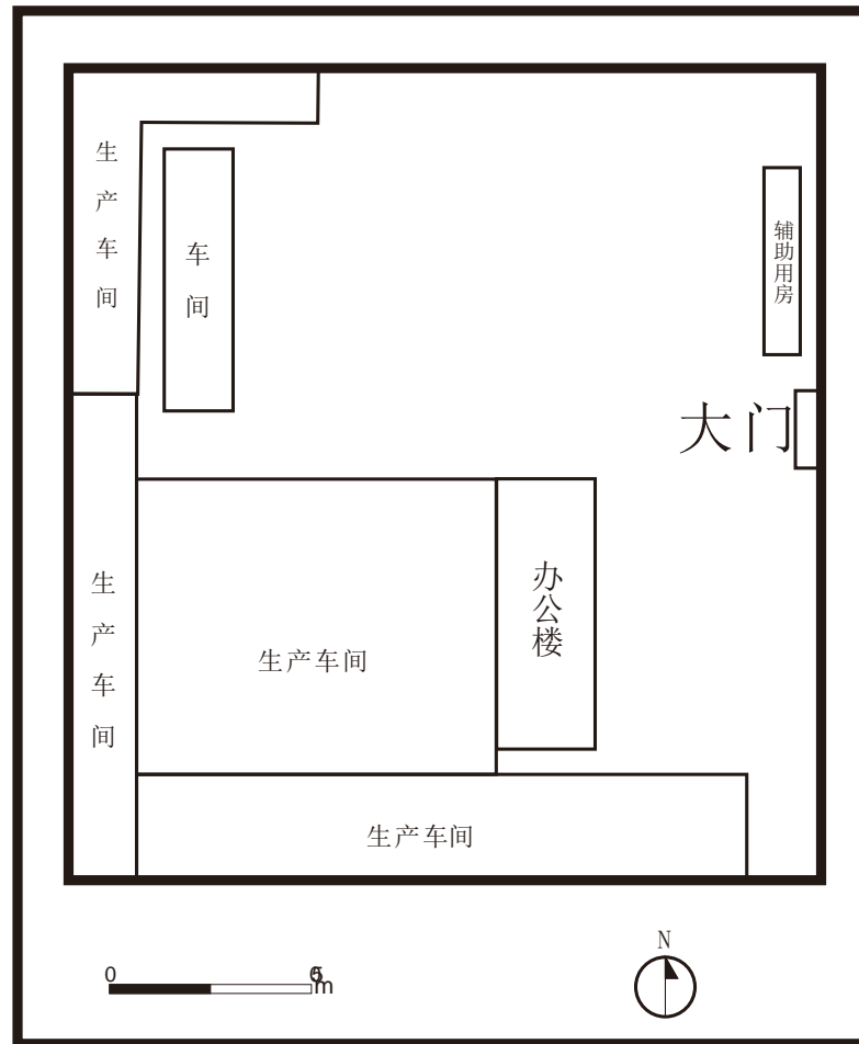
附图2 本项目全厂平面布置图
