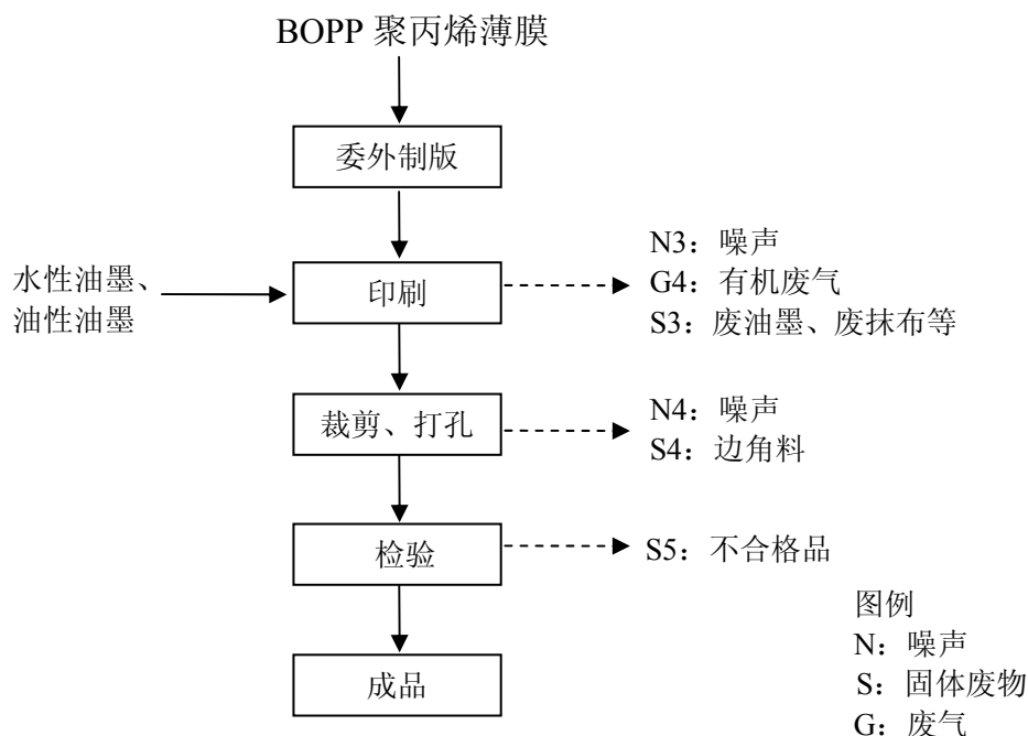
图 2.2-2 印刷生产工艺流程图
