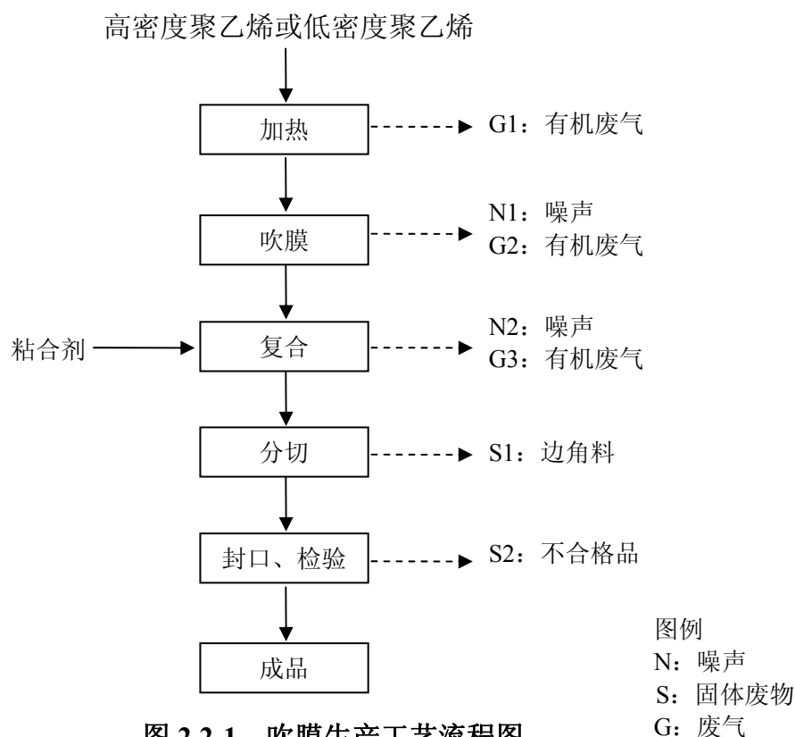
图 2.2-1 吹膜生产工艺流程图
