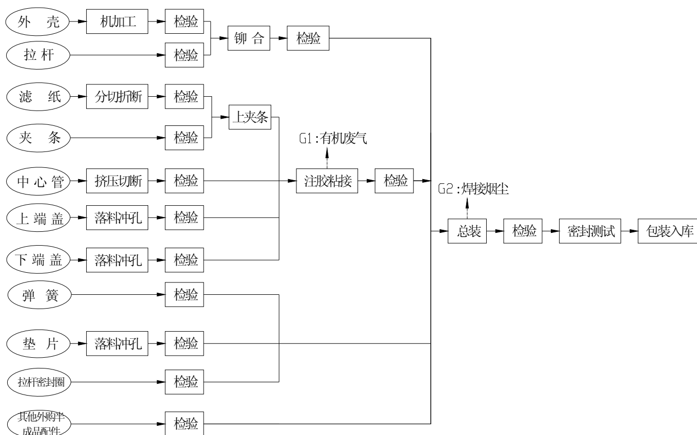
图 2.2-1 柴油滤清器和机油滤清器生产工艺流程图
