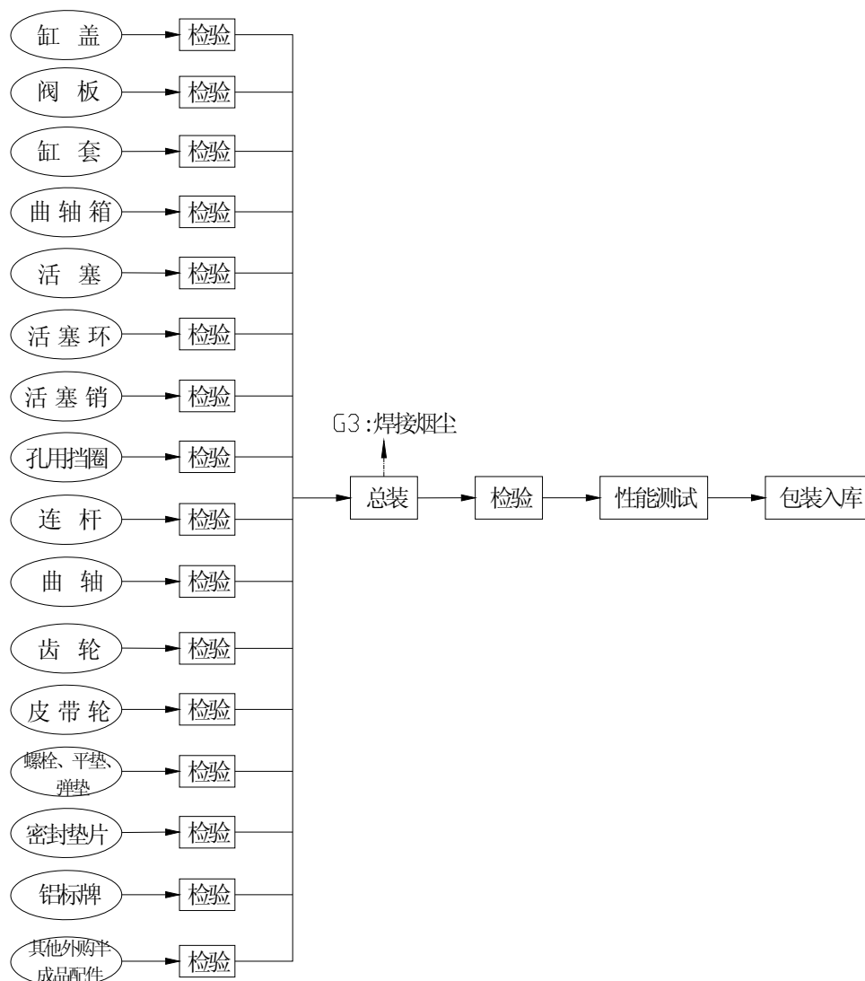
图 2.2-2 车用空压机生产工艺流程图
