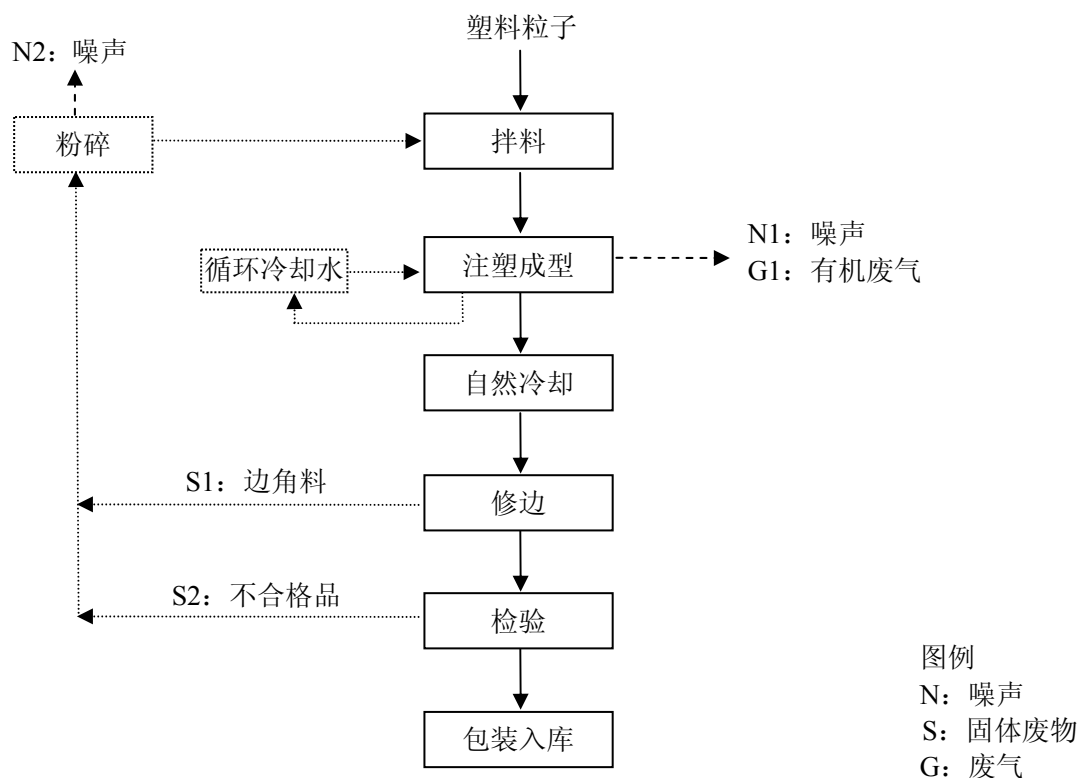
图 1 建设项目生产工艺流程图
