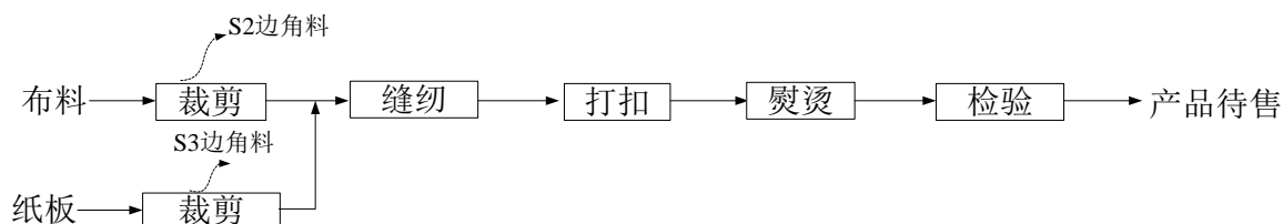
图2.2-2 储物盒生产工艺流程框图及主要产污环节图
