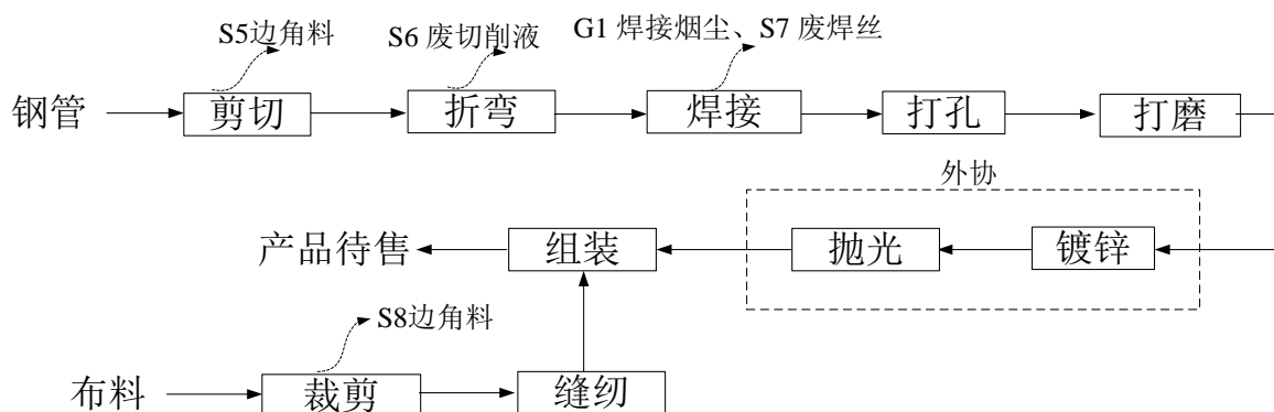
图2.2-4 衣柜生产工艺流程框图及主要产污环节图
