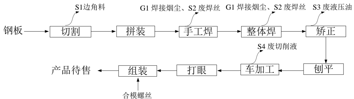
图2.2-1 管桩钢模生产工艺流程框图及主要产污环节图
