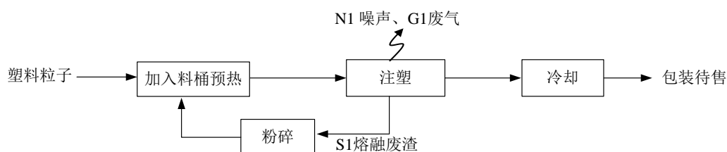
图2.2-2 充电器外壳生产工艺流程图及主要产污环节图
