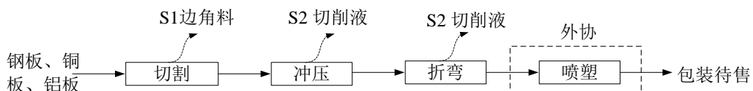
图2.2-1 电器配件生产工艺流程框图及主要产污环节图
