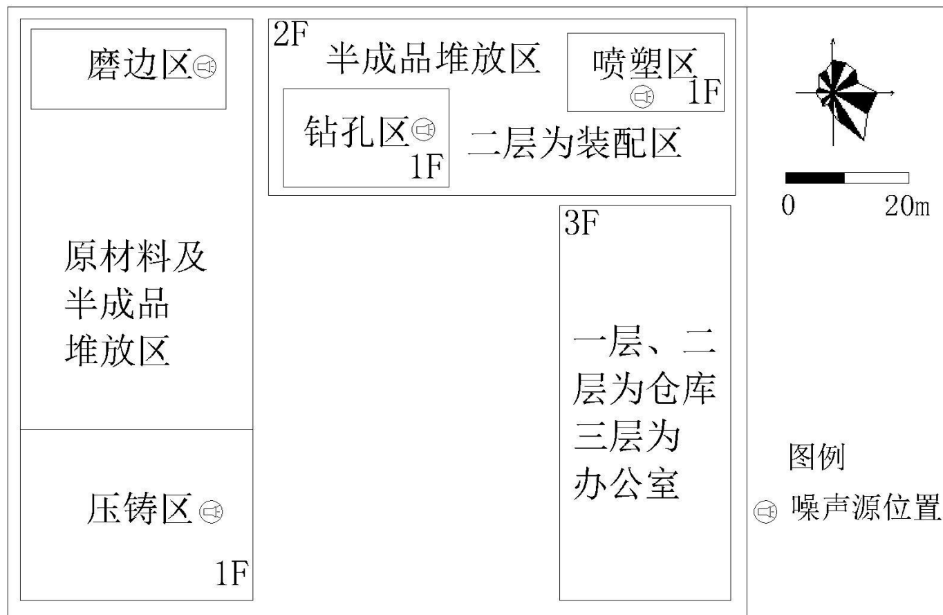
附图3 本项目厂区平面布置图
