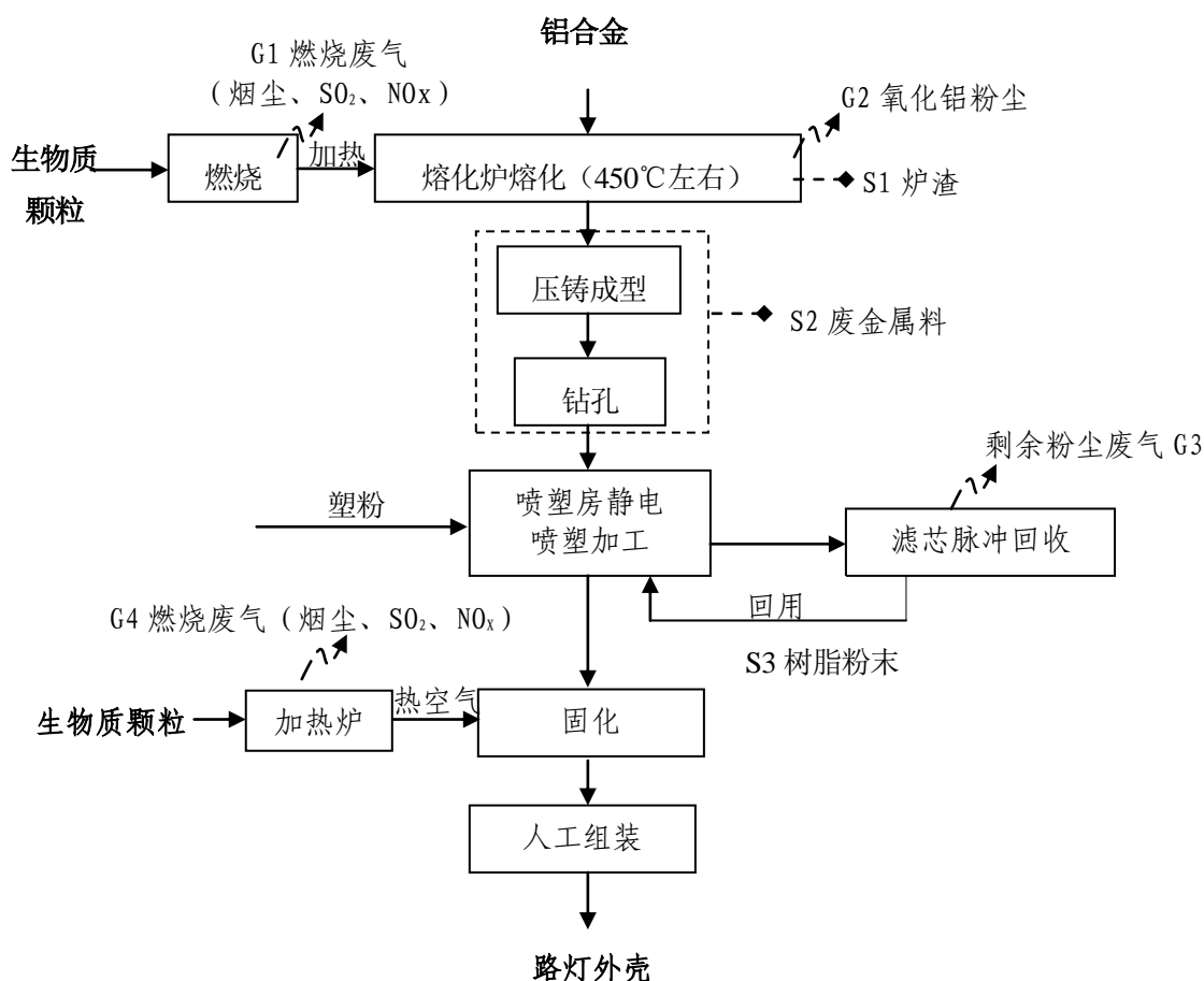
图 2.2-1 路灯外壳生产工艺及产污环节示意图
