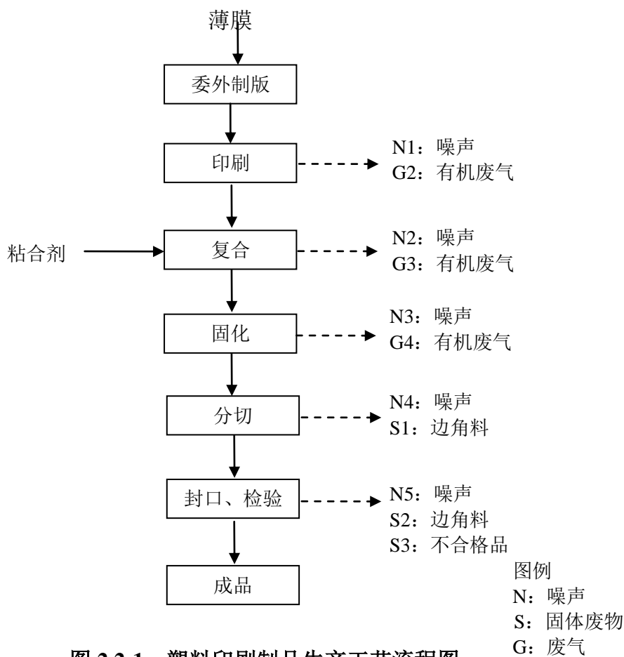
图 2.2-1 塑料印刷制品生产工艺流程图
