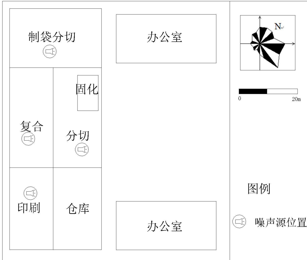
附图3 本项目厂区平面布置图
