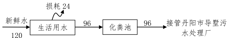
图 2.2-2 本项目用水排水平衡图 (t/a)
