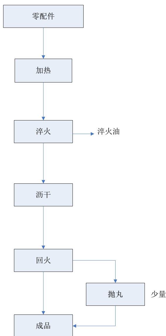
图 2.2-1 本项目旅游用品生产工艺流程及产污环节框图 工艺说明：
