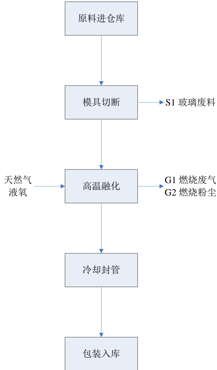
图 2.2.1-1 本项目拉链生产工艺流程框图及主要产污环节图
