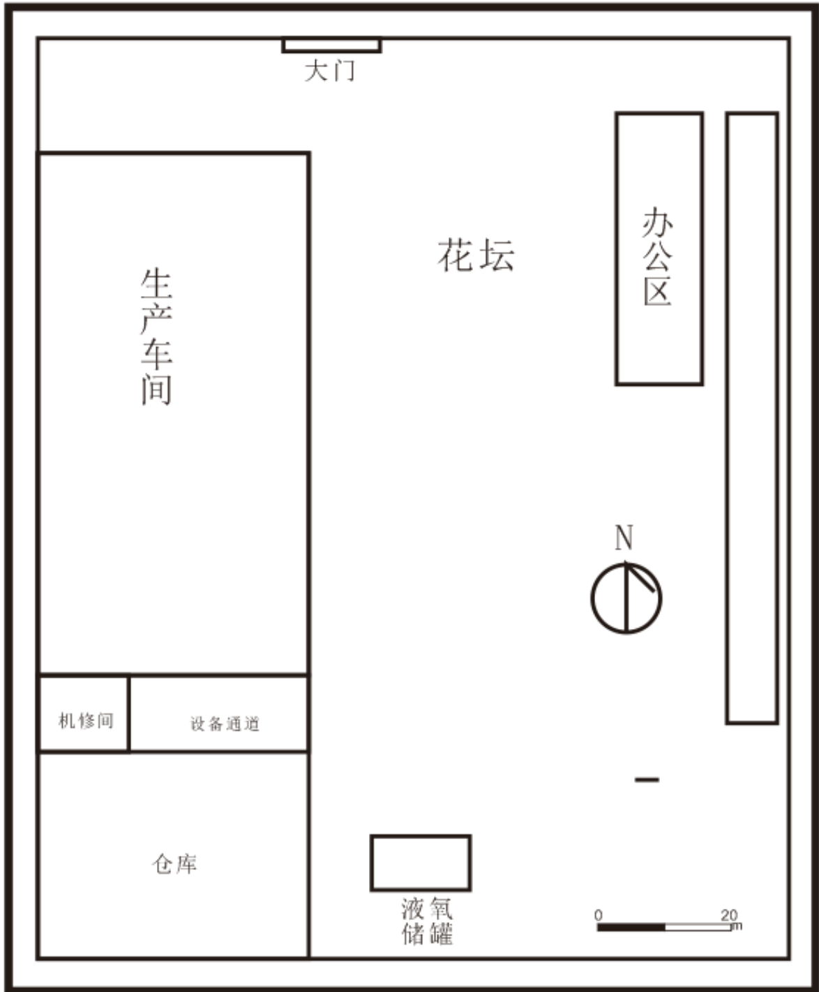
附图3 建设项目全厂平面布置示意图
