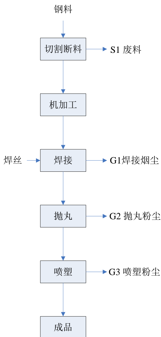
图 2.2-1 生产工艺流程图
