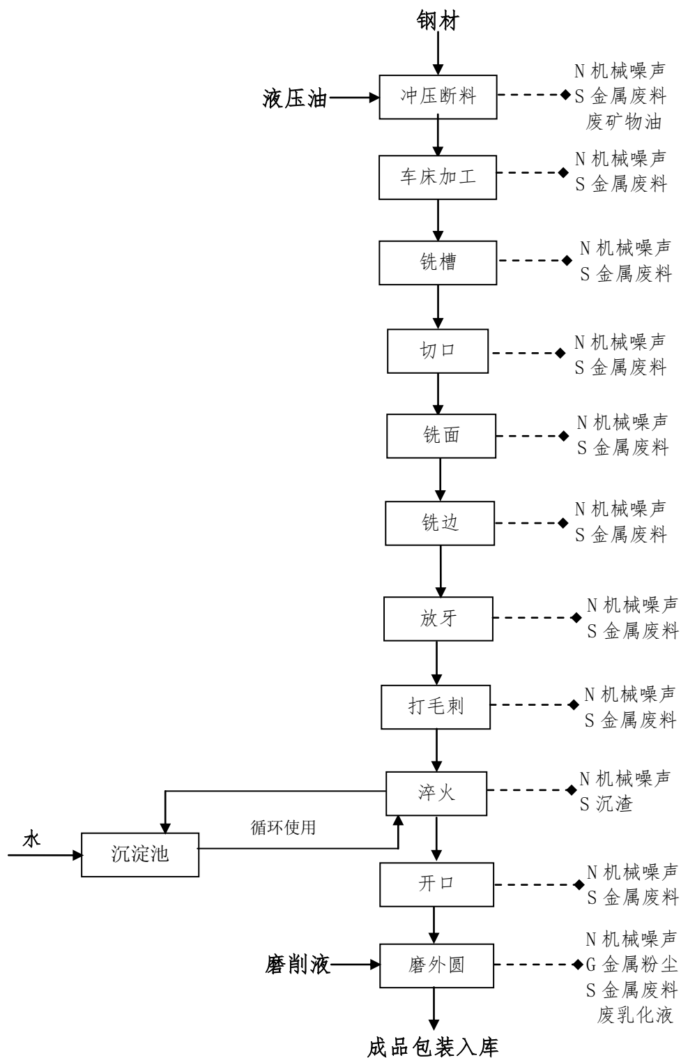
图 2.2-1 本项目合金锯片生产工艺流程及产污环节图
