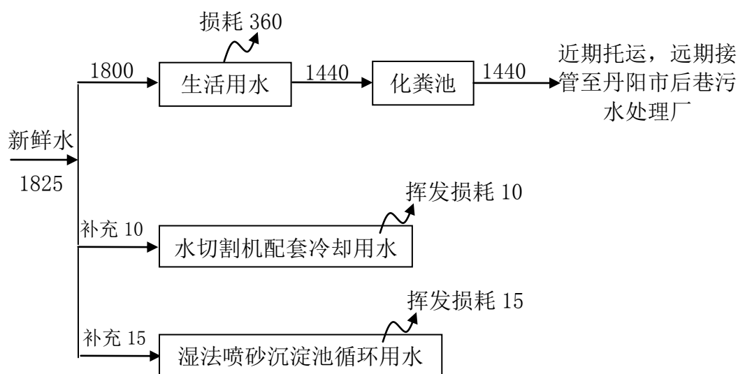
图 2.2-2 本项目用水排水平衡图 (t/a)
