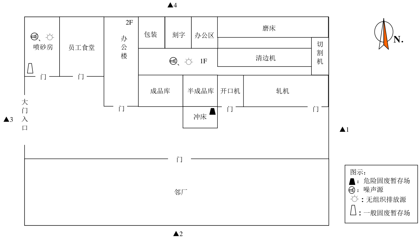
附图2 本项目厂区平面布置图
