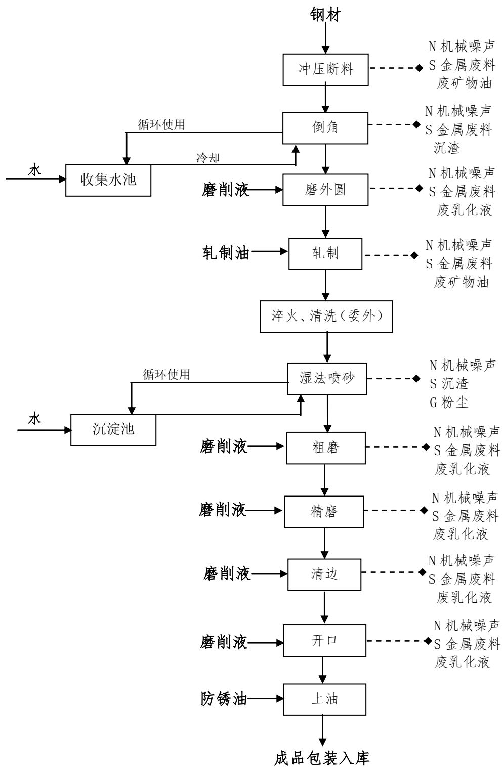
图 2.2-1 本项目合金锯片生产工艺流程及产污环节图
