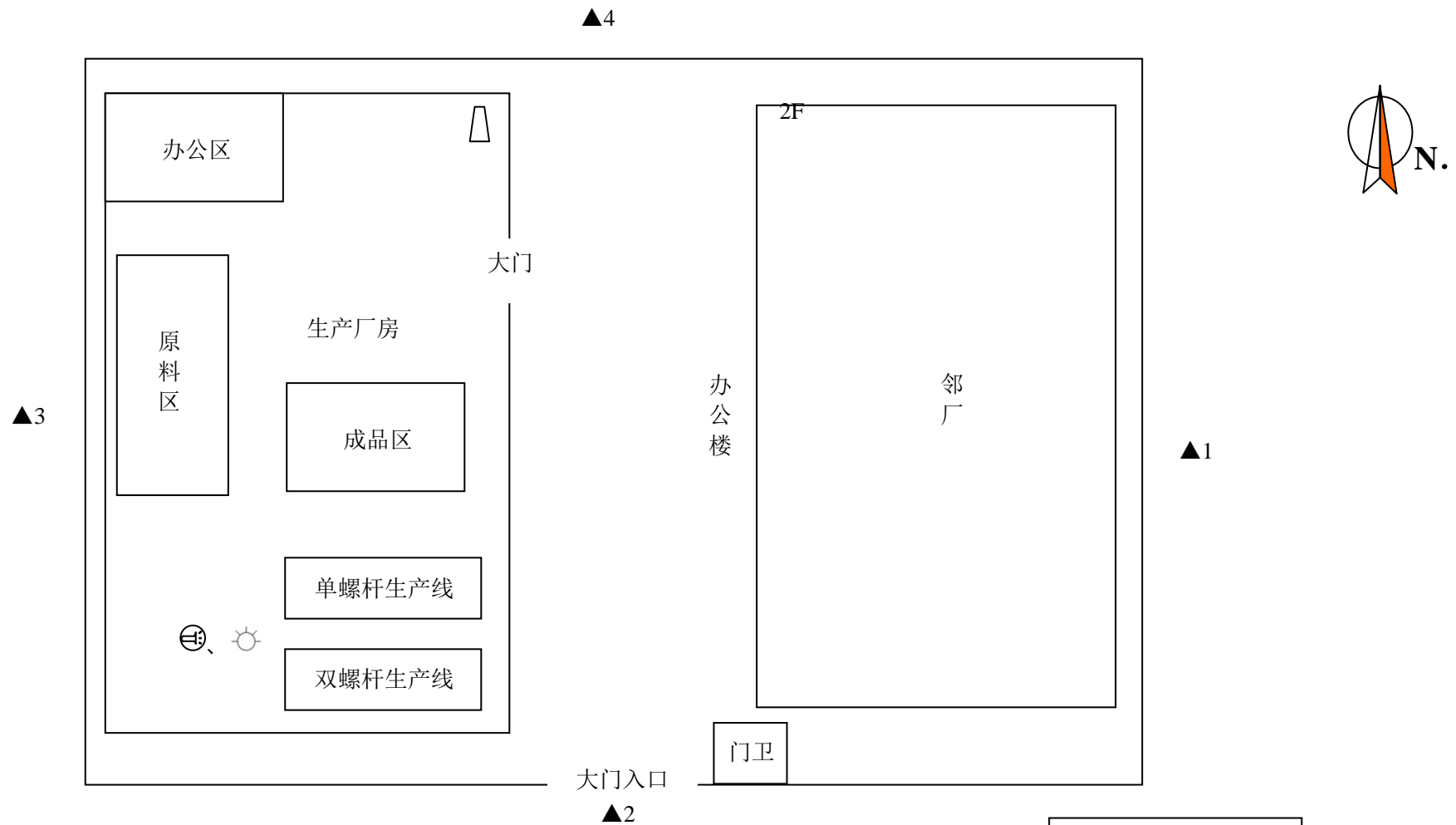
附图2 本项目厂区平面布置图（附噪声监测点位图）
