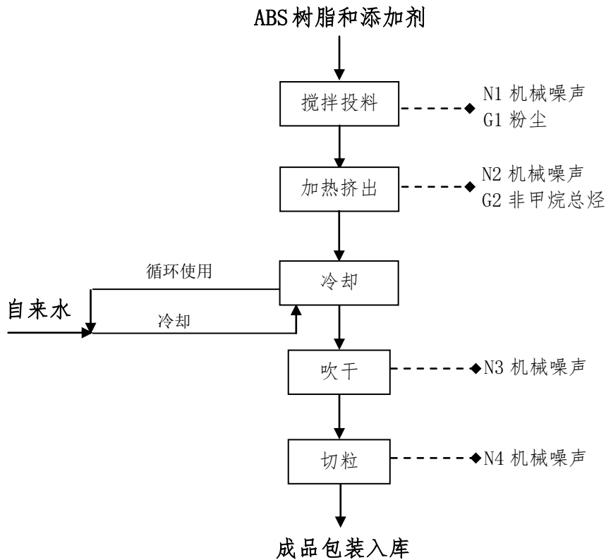
图 2.2-1 本项目改性塑料粒子生产工艺流程及产污环节图
