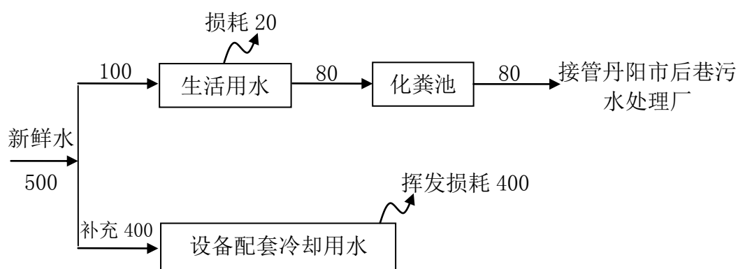
图 2.2-2 本项目用水排水平衡图 (t/a)
