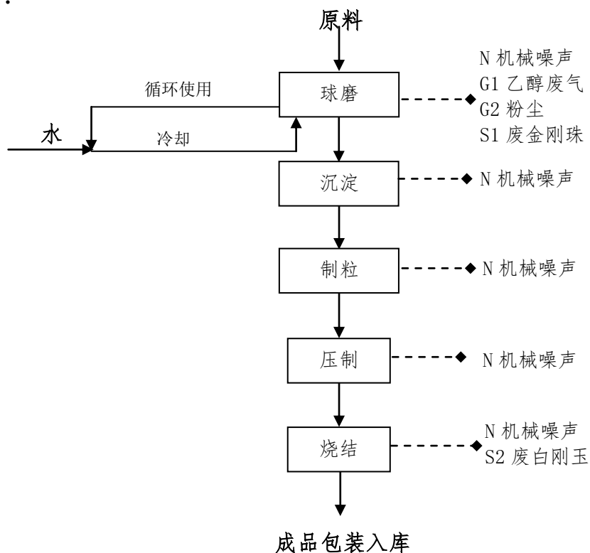
图 2.2-1 本项目（碳钨特钢）合金刀头生产工艺流程及产污
