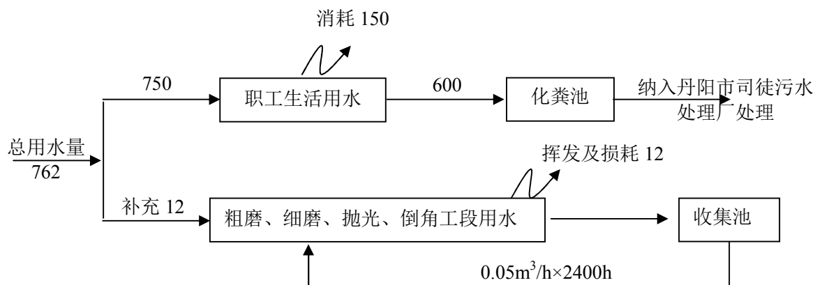
图 2 本项目水量平衡图（单位：m 3 /a）
