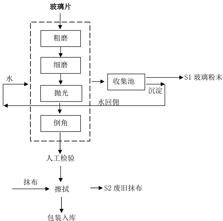
图1 本项目眼镜镜架生产工艺流程及产污环节 工艺说明：
