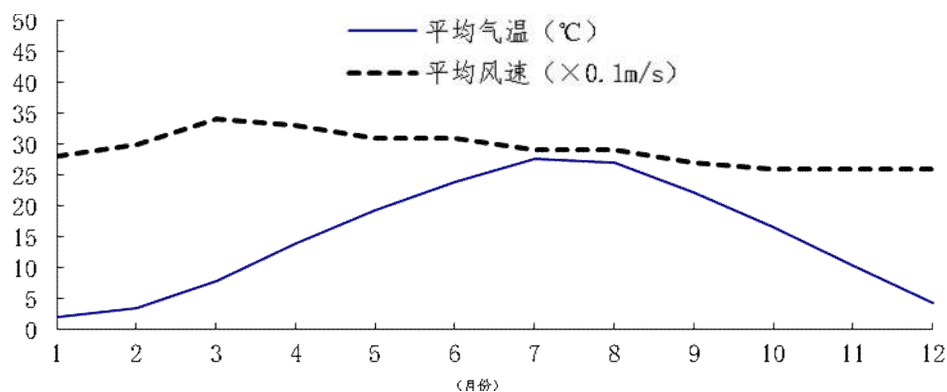
图 4 丹阳市风速、气温年变化曲线
