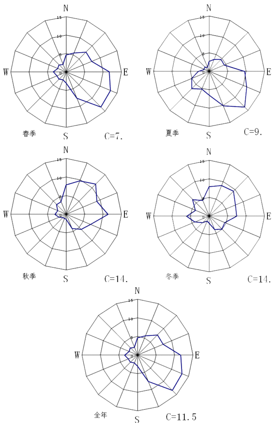
图 5 丹阳市风向频率玫瑰图
