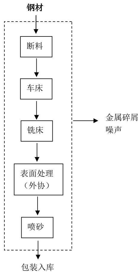
图 1 生产工艺及产污环节图
