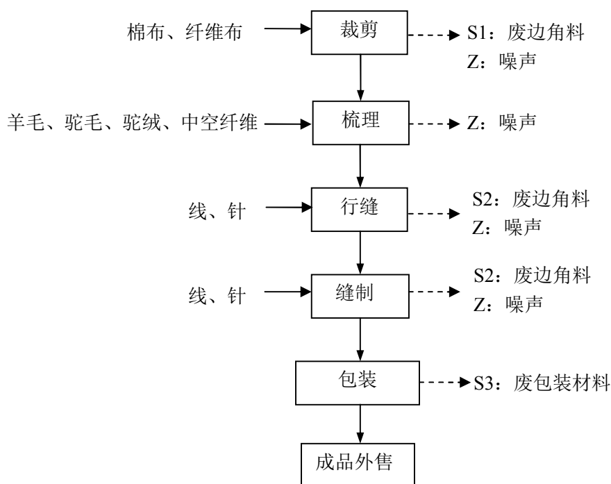
图 2.2-1 被子、枕头及床上四件套生产工艺流程及产污环节
