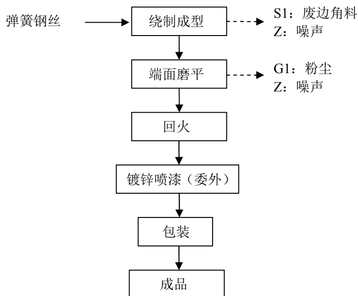
图 2.2.1-2 弹簧生产线生产工艺流程框图及主要产污环节图
