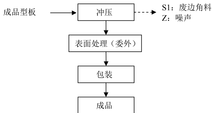
图 2.2.1-1 冲压件生产线生产工艺流程框图及主要产污环节图
