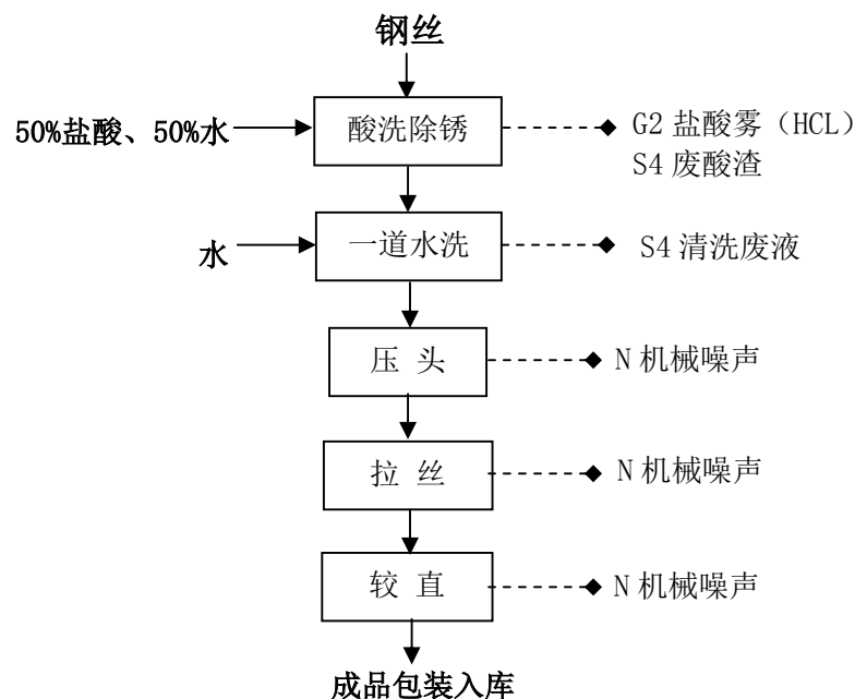
图 2.2-1 本项目钢丝生产工艺流程及产污环节图
