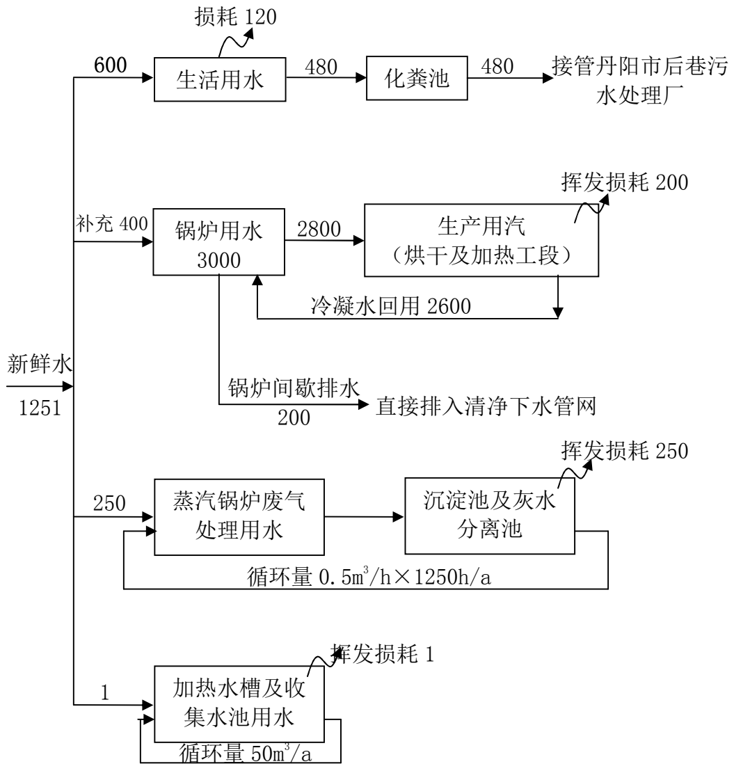
图 2.2-2 本项目用水排水平衡图 (t/a)
