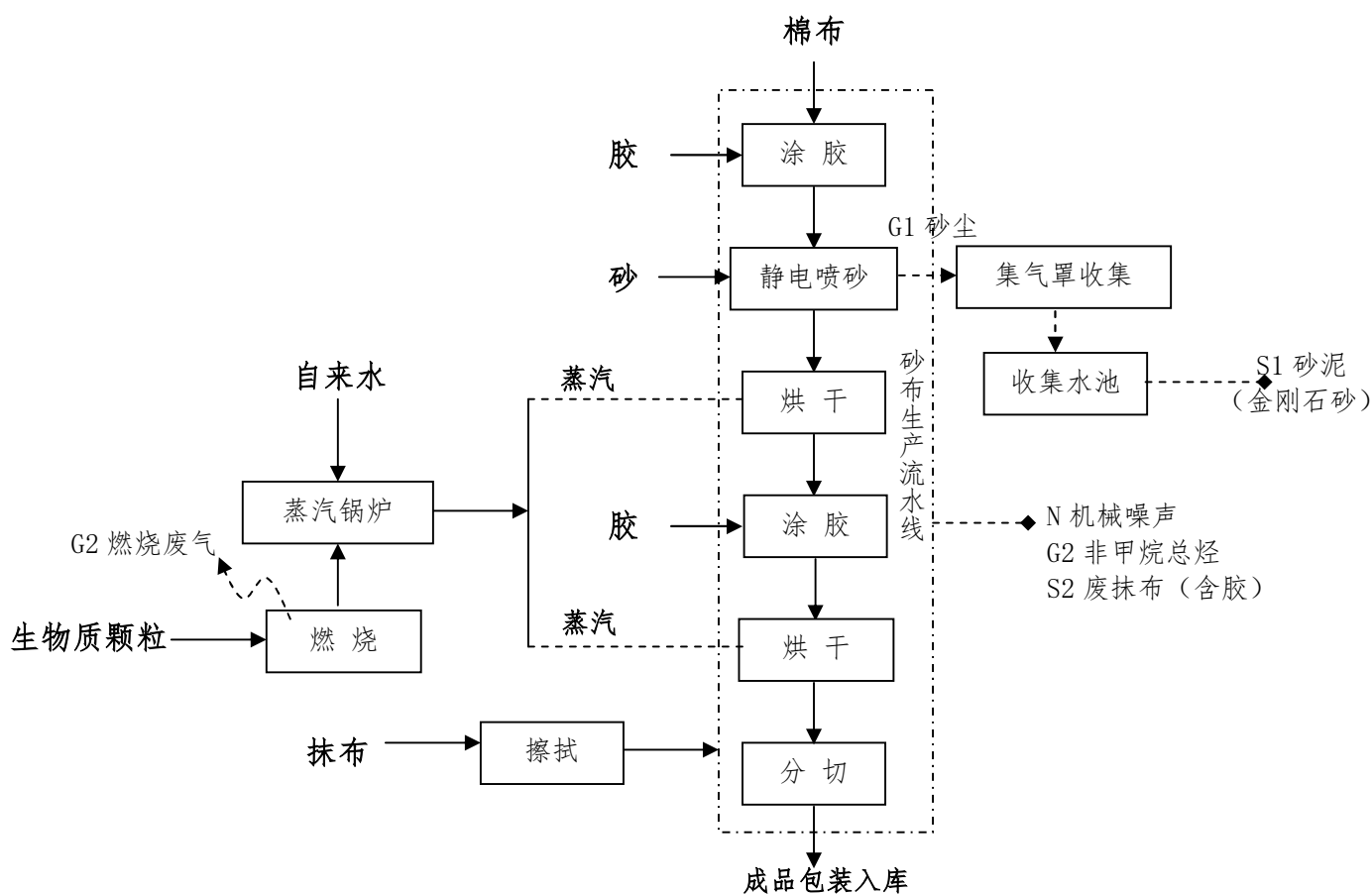
图 2.2-1 本项目砂布生产工艺流程及产污环节图
