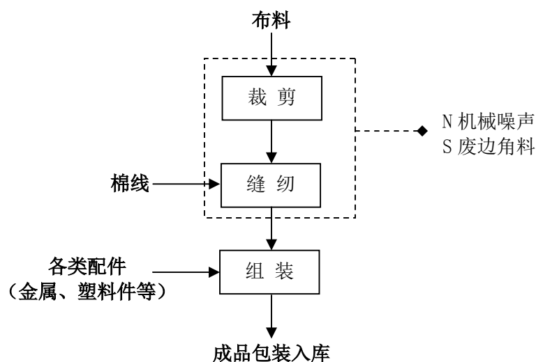
图 2.2-1 本项目旅游用品生产工艺流程及产污环节框图
