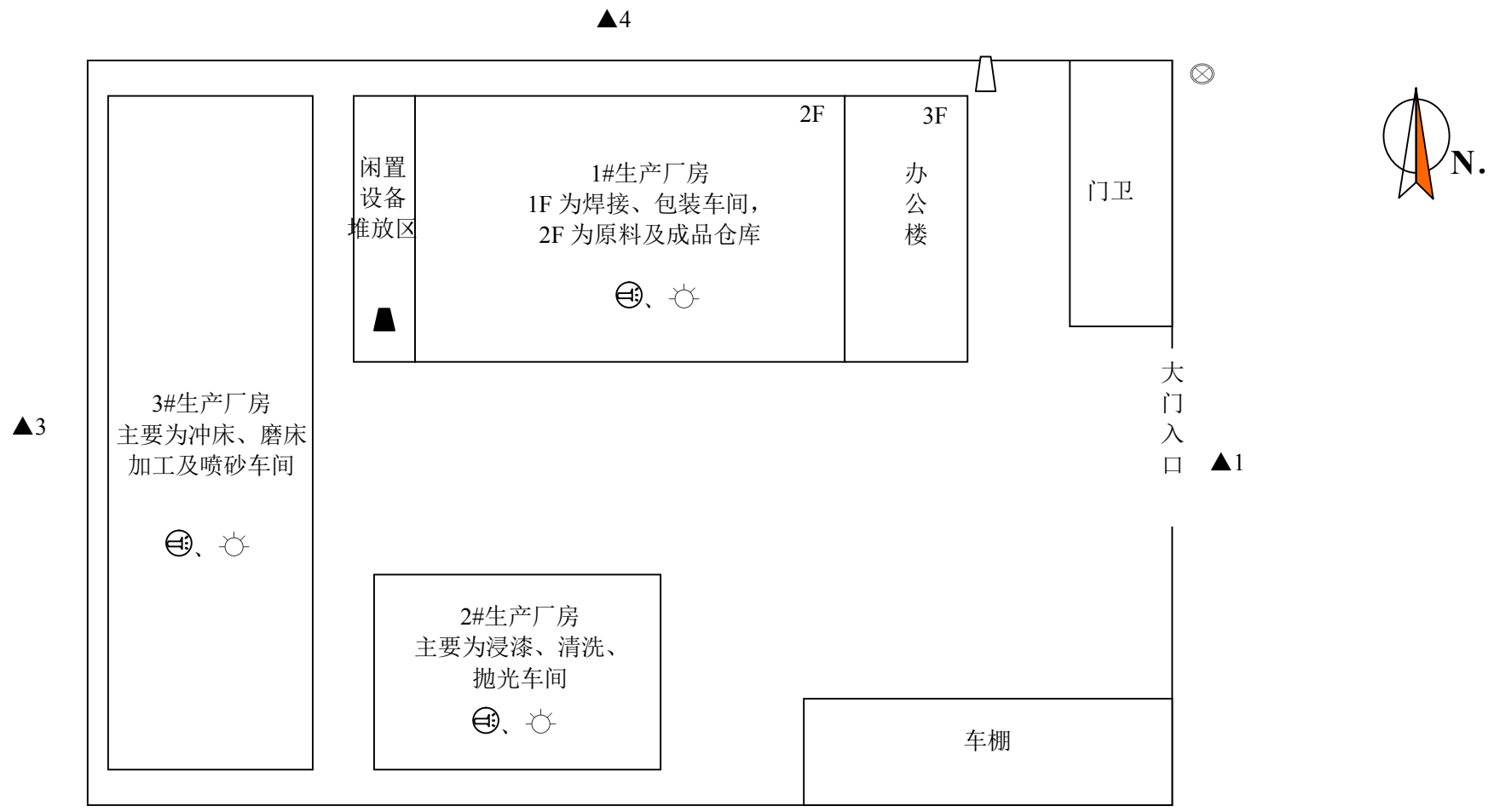
附图2 本项目厂区平面布置图
