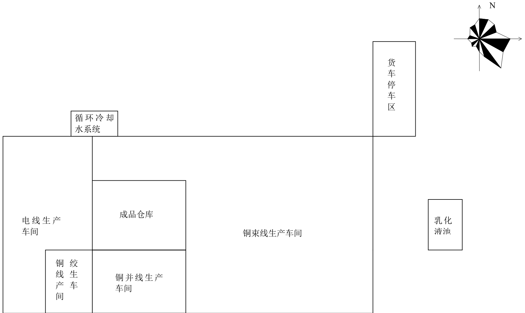
附图 3 项目平面布置示意图
