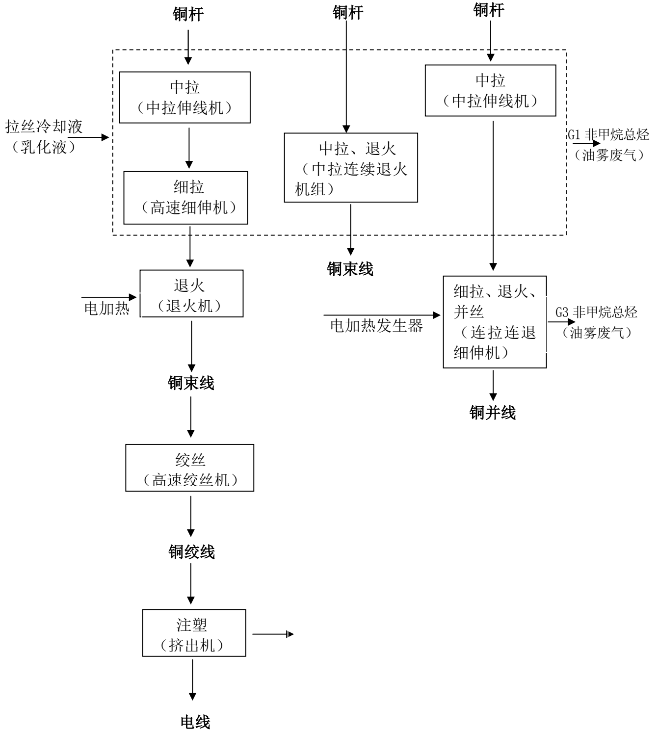
图 1 生产工艺及产污环节图
