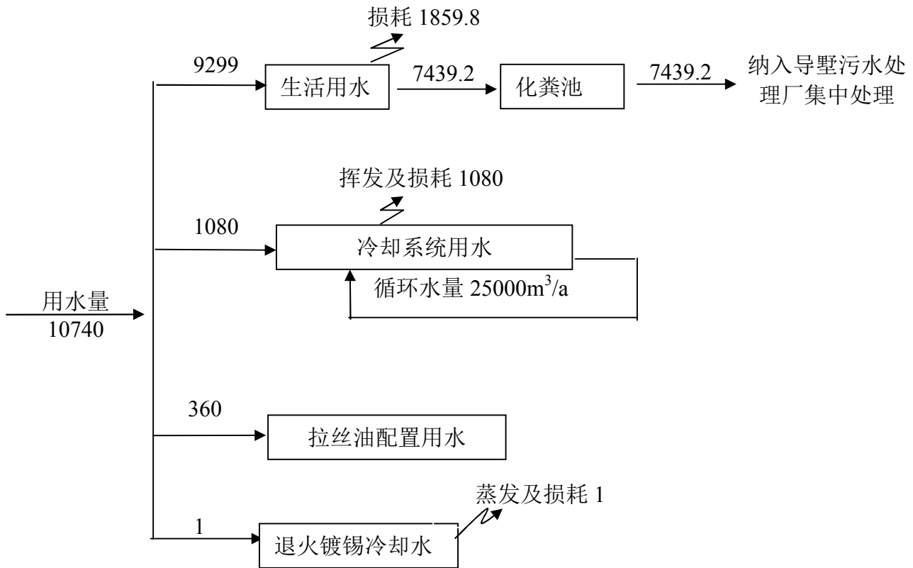
图 2 该项目水量平衡图（单位：m 3 /a）
