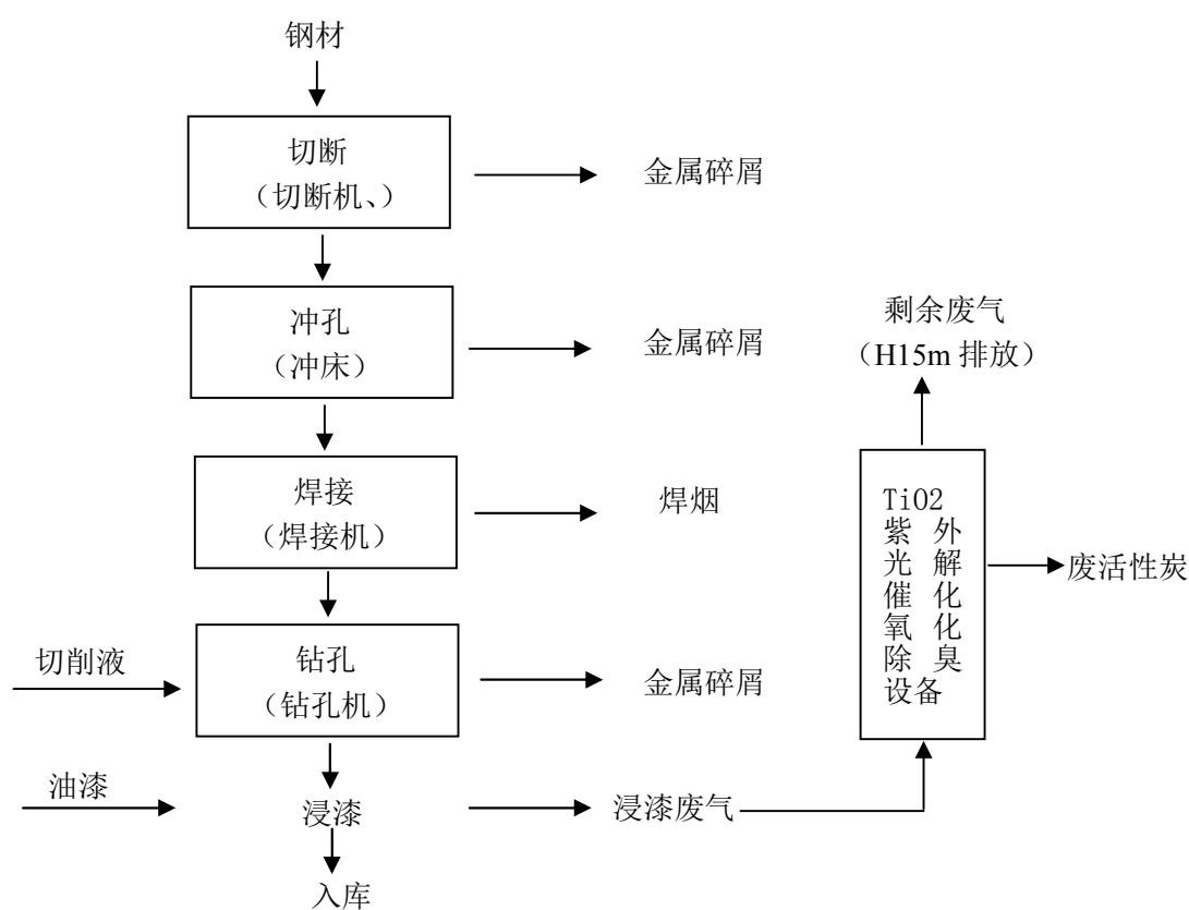
图 1 生产工艺及产污环节图
