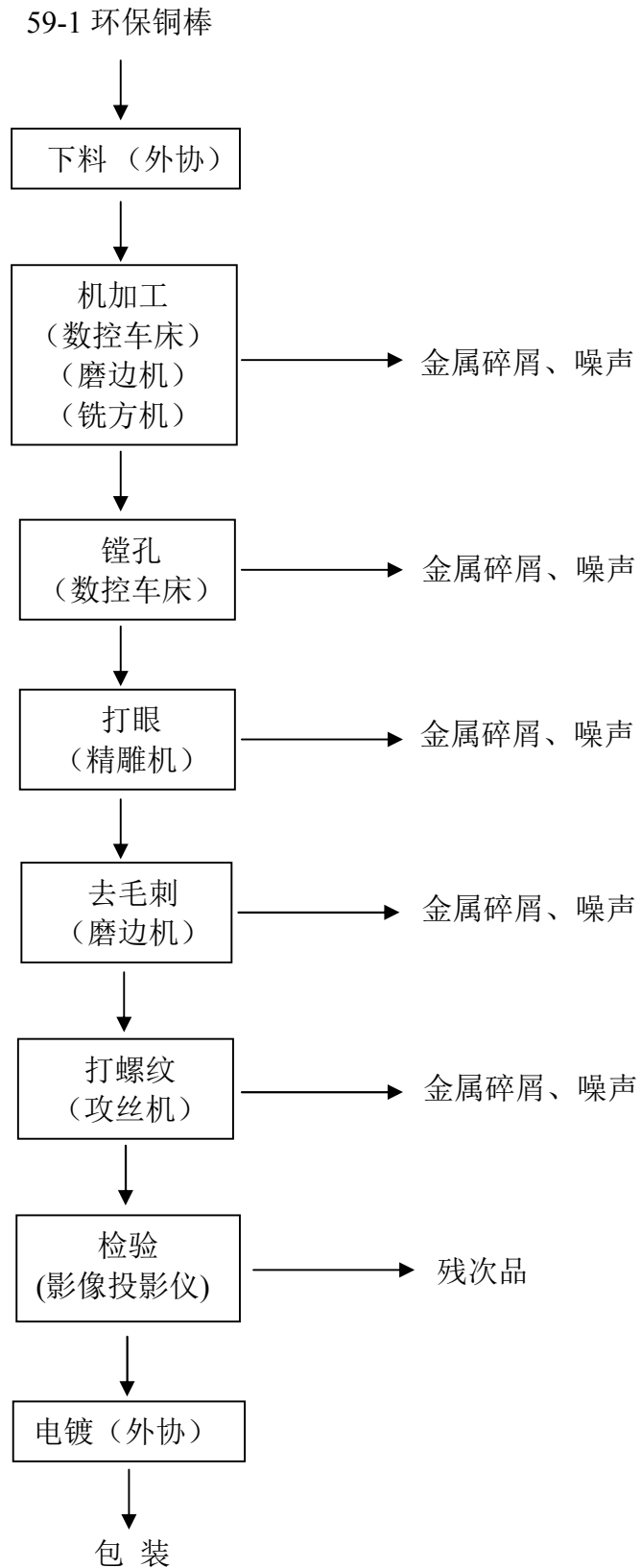
图 1 生产工艺及产污环节图
