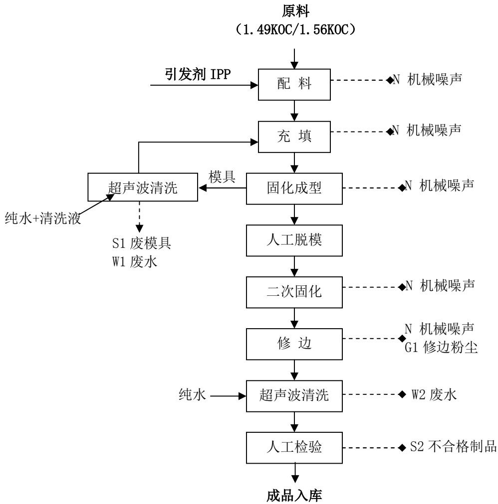
图 2.2-1 光学树脂镜片生产工艺流程及产污环节框图
