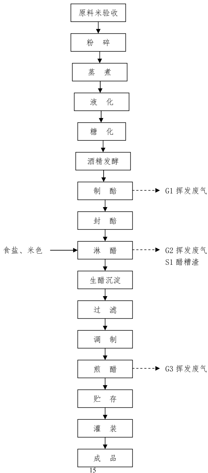
图 2.2-1 项目工艺流程及产污环节框图
