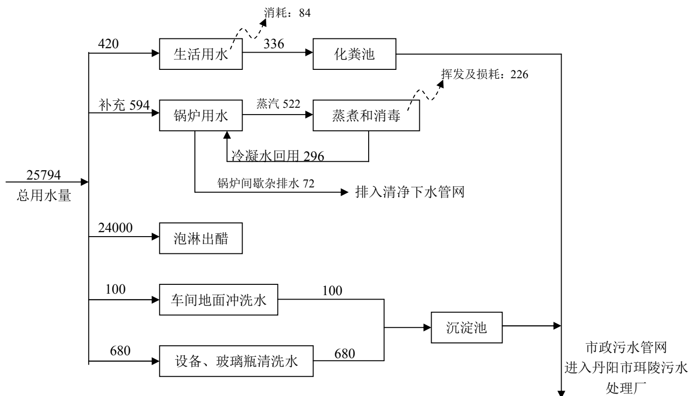
图 2.1-2 项目水量平衡图 (单位: m³/a)
