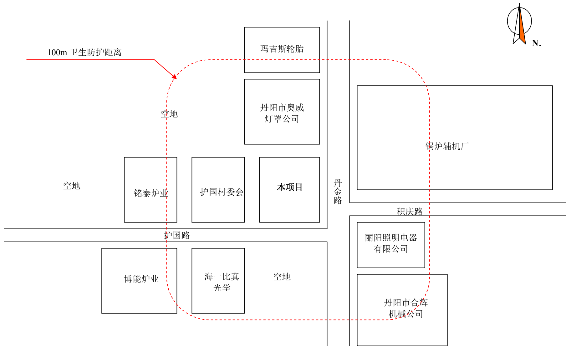
附图3 项目厂界周围环境简况图
