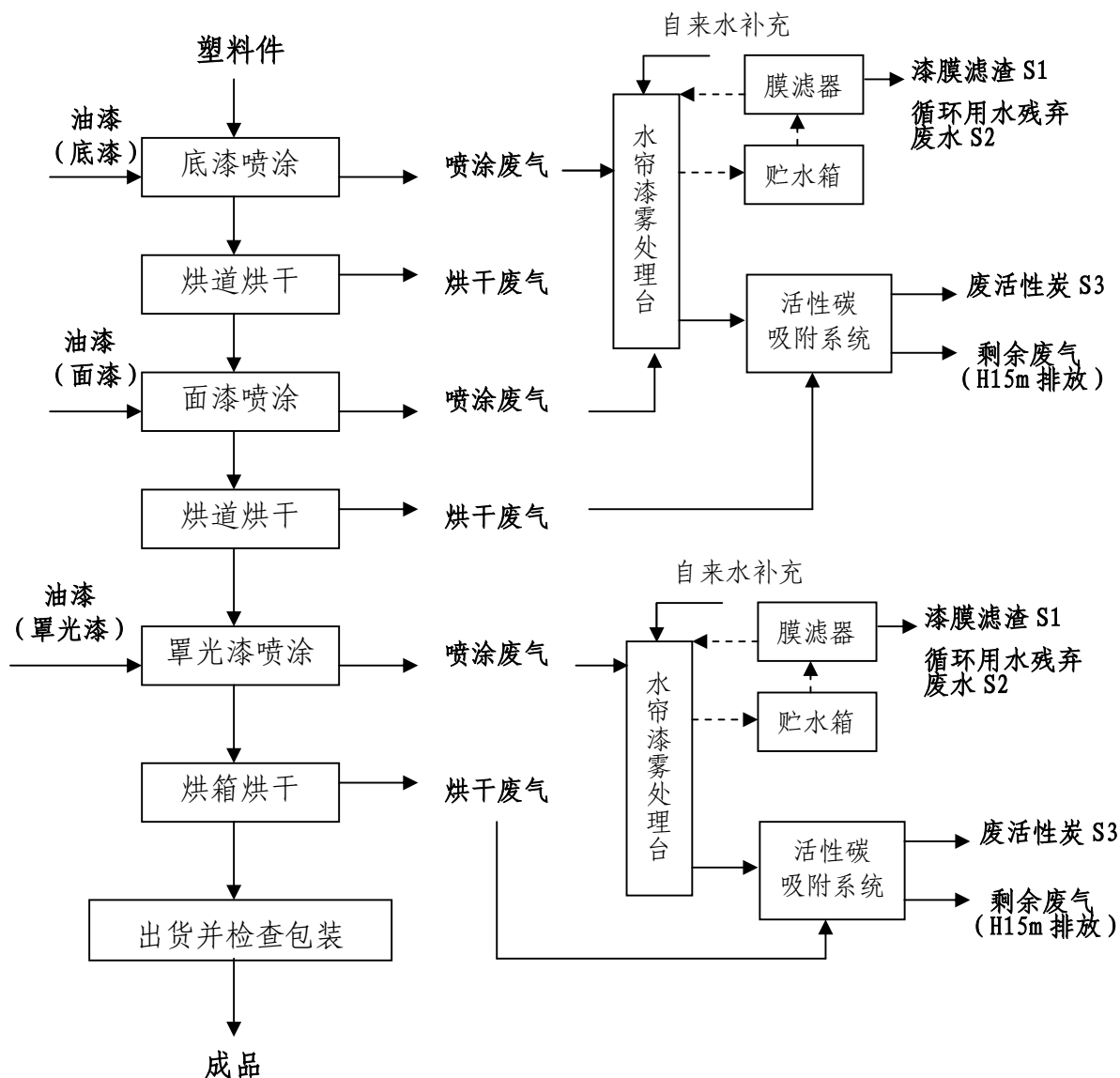
图 2.2.1-1 本项目涂装流水线生产工艺流程框图及主要产污环节图
