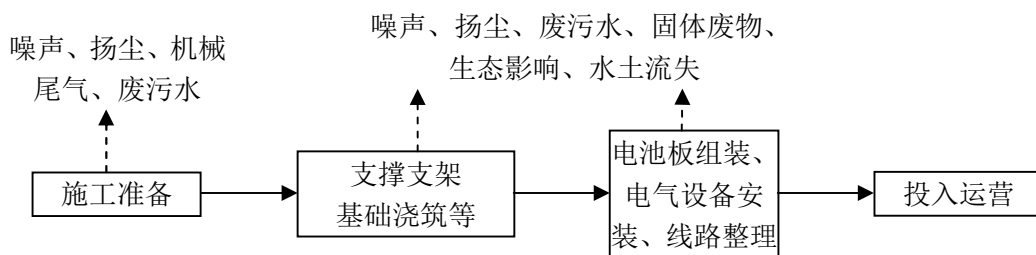
图 1 项目光伏电场施工期主要工艺流程及产污环节
