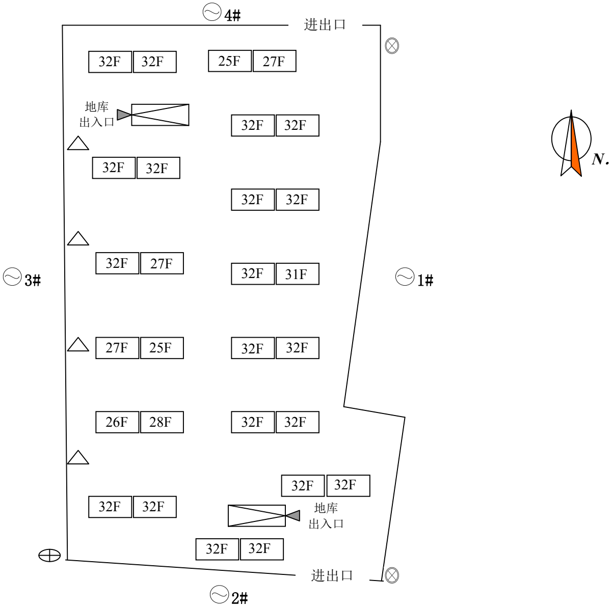
附图 2 本项目平面布置图（附噪声监测点位）
